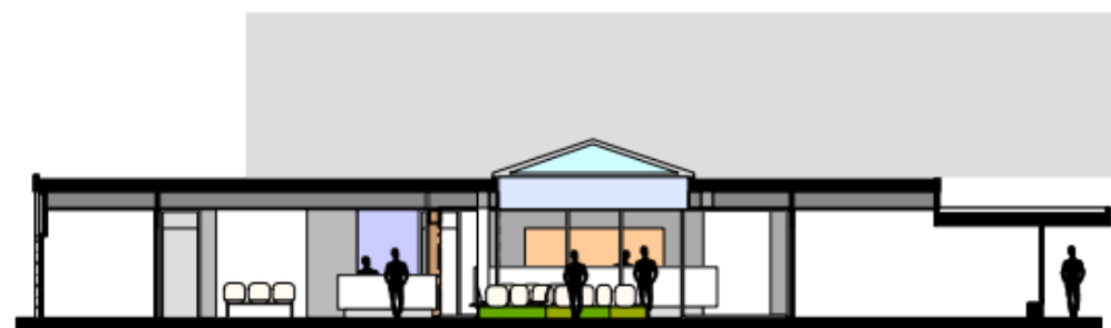
doorsnede A-A
